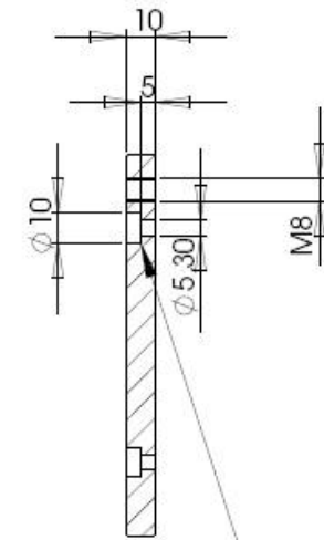
SCHNITT T-T
