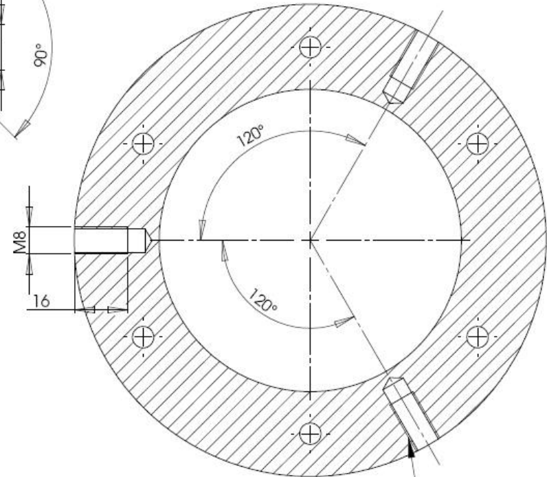
SCHNITT U-U MAßSTAB 1 : 1
