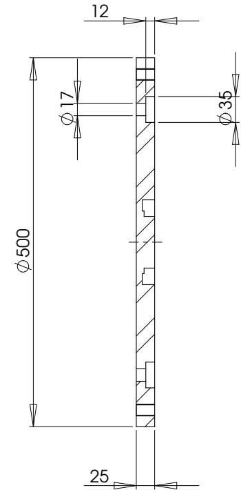
SCHNITT R-R MAßSTAB 1 : 5
